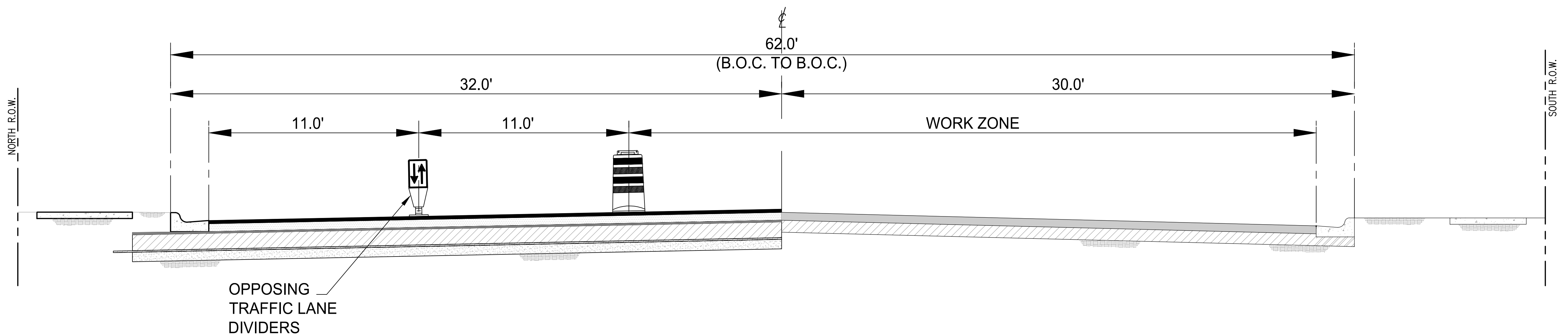
GREENWOOD TRAFFIC CONTROL PHASE II SCALE: N.T.S.
