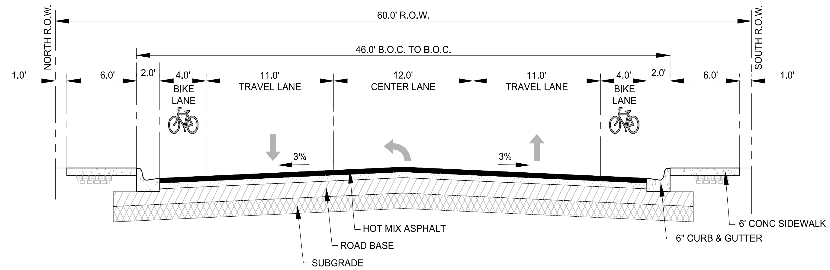
PROPOSED ROADWAY (STA. 0+00 THRU STA. 19+34)
